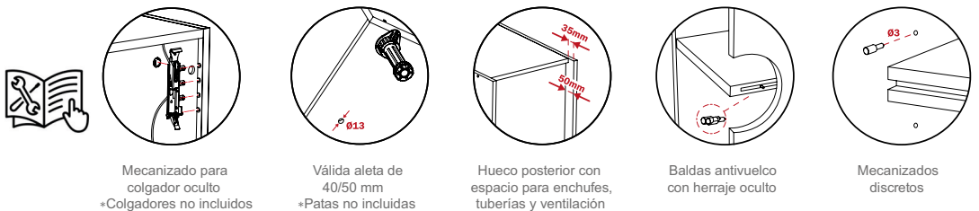
Mecanizado para colgador oculto *Colgadores no incluidos
